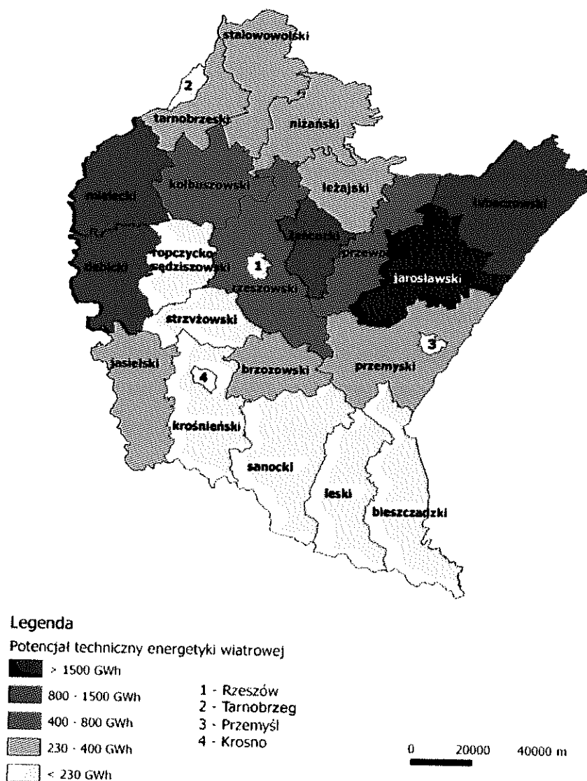
Rys. 4 Potencjał techniczny energetyki wiatrowej
