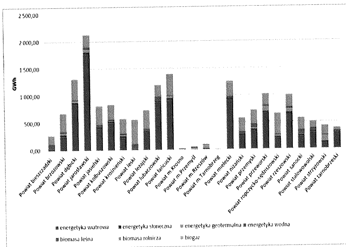
Wyk. 3 Potencjał techniczny OZE dla sektora energetycznego w powiatach województwa podkarpackiego GWh
